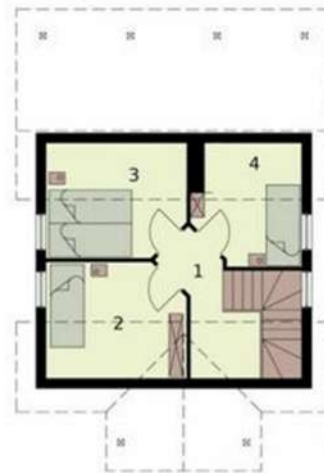
Osnova potkrovlja
