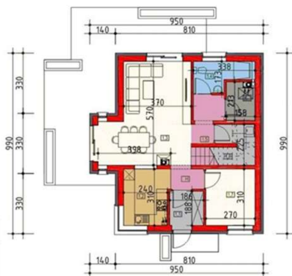
Osnova prizemlja
