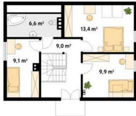
Osnova potkrovlja
