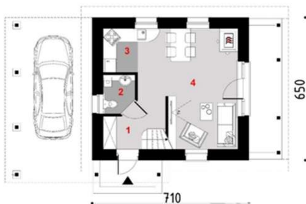
Osnova prizemlja
