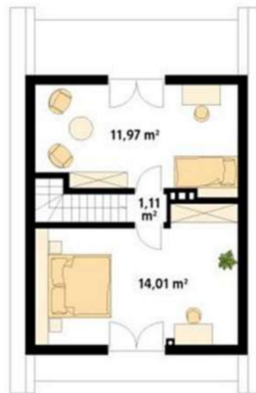
Osnova potkrovlja
