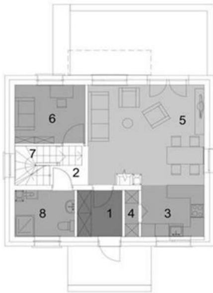
Osnova prizemlja
